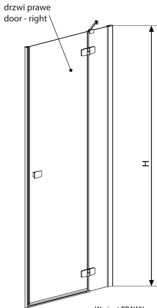
Wariant PRAWY Variant R
